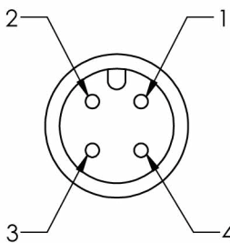
4 PIN M12
